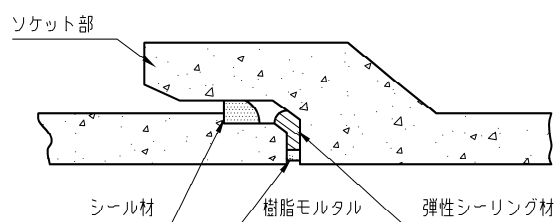
図 3.3.2.1-1 継ぎ手部止水方法
