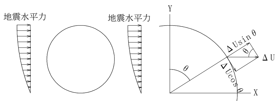
図 2.2.8.1-9 地震水平力
