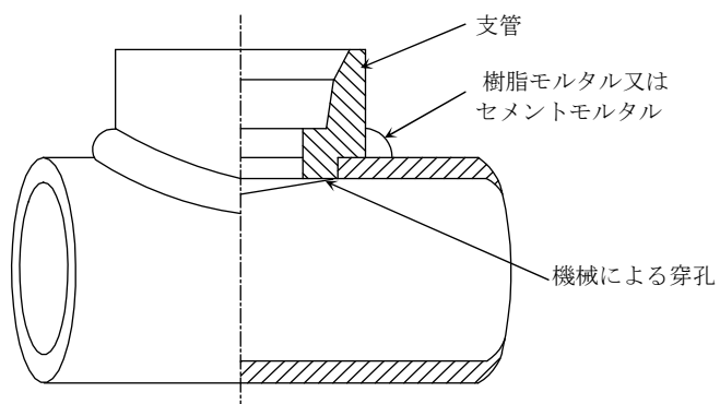
図 3. 1. 4. 5-1 支管の取り付け方法
