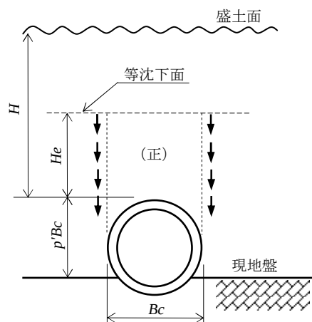
図 2.2.3.1.1-3 正の突出型
