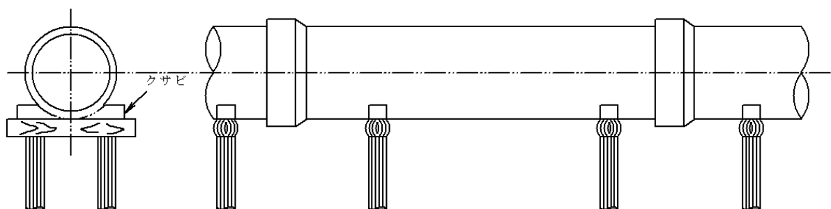
図 3.1.3.1-5 鳥居基礎（くい打ち基礎）
