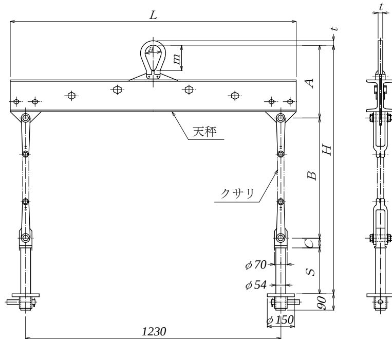
図 3.2.6.1-2 吊具の一例
