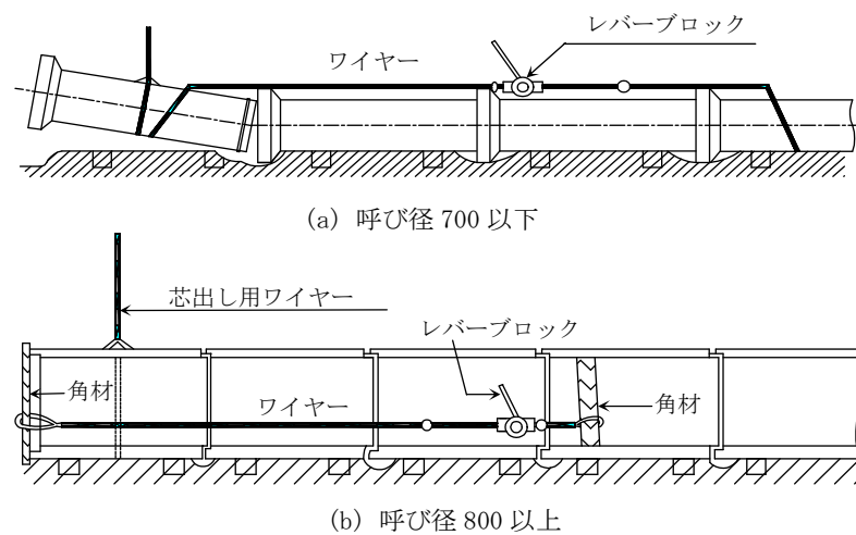
図 3.1.4.2-3 接合方法
