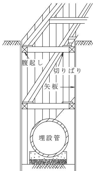
図 3.1.2.2-1 木矢板工法
