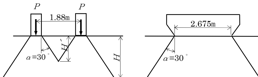
図 2.2.2.3-2 荷重分布図
