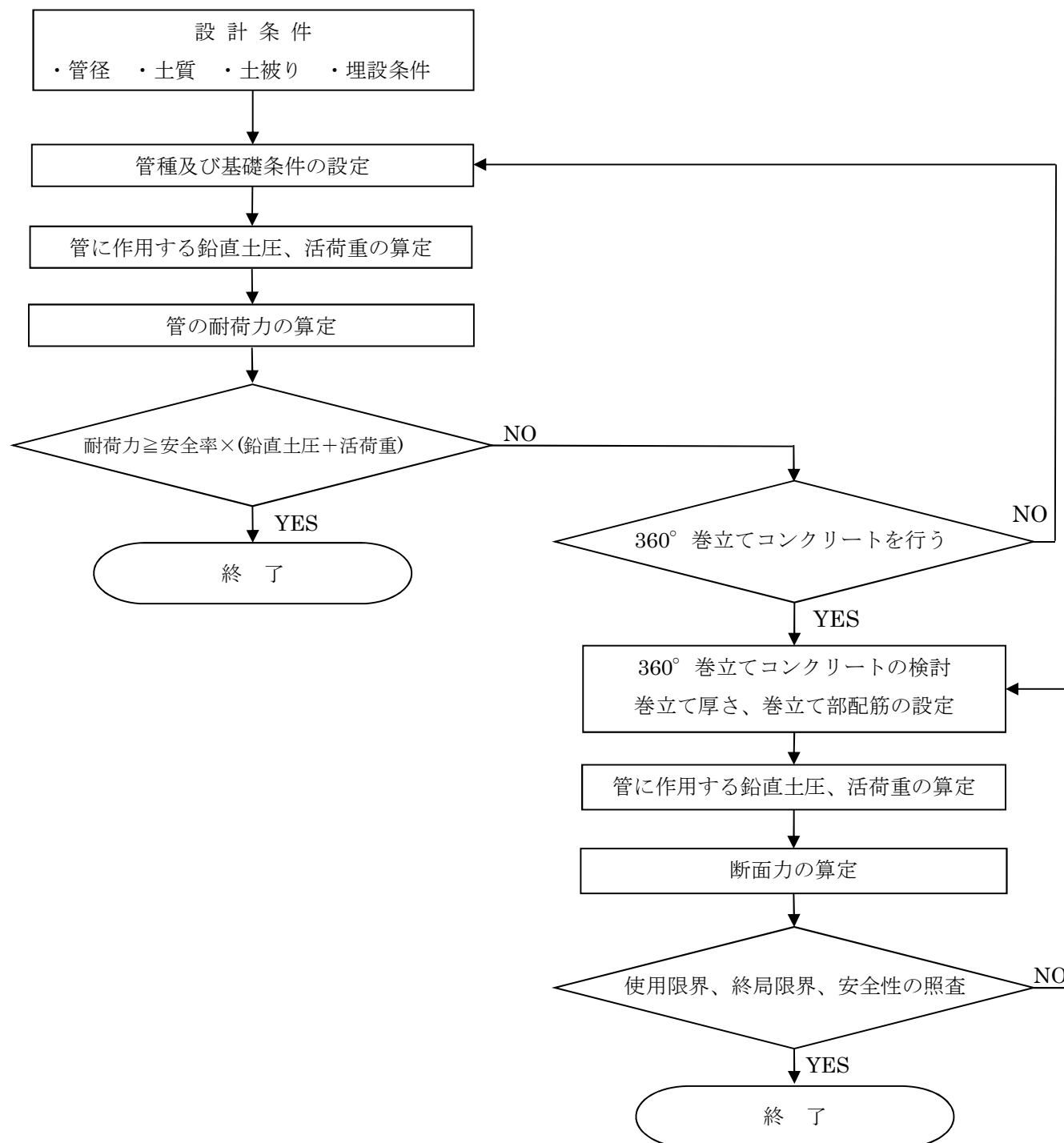
図 2.2.4-1 開削管の設計フローチャート
