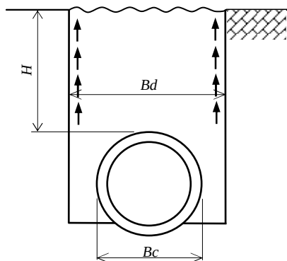
図 2.2.3.1.1-2 溝 型
