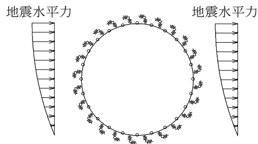
図 2.2.8.1-5 地震水平力の分布モデル
