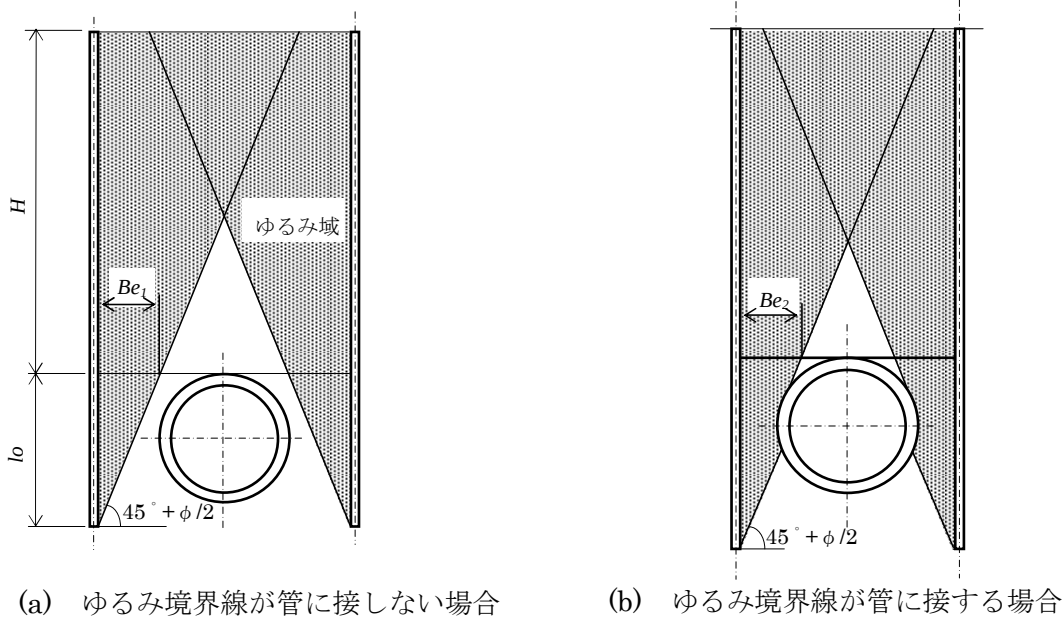
図 2.2.3.1.2-4 ゆるみ幅 B_e
