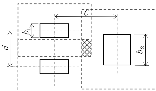
図 2.2.2.2-4 前後輪荷重分布
