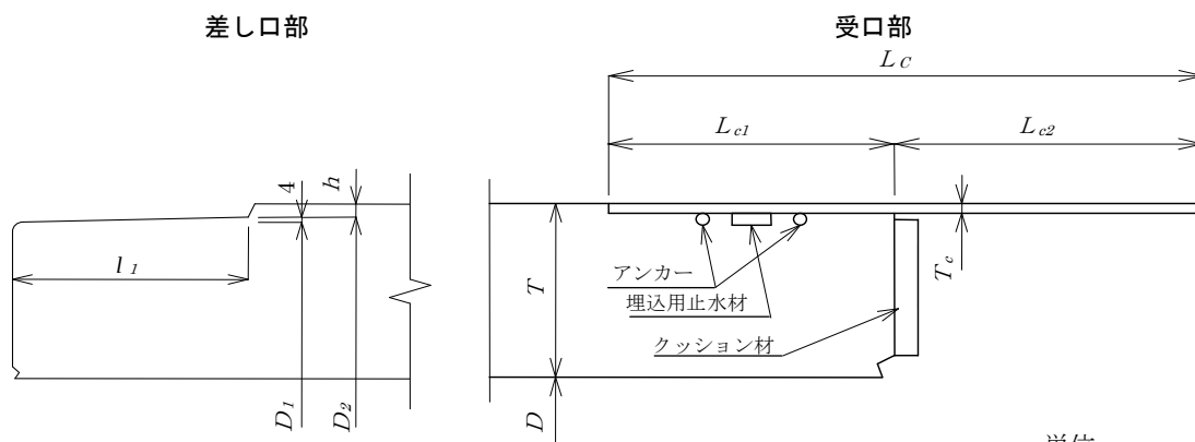
継手部詳細図
