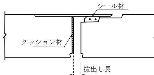
図 1.4.4-1 拔出し長
