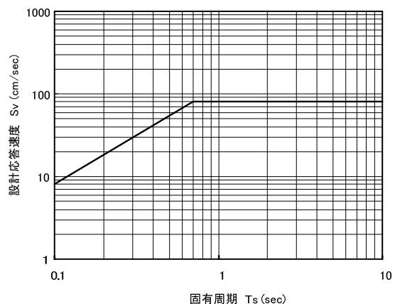
図 2.2.8.1-7 レベル 2 地震動 設計応答速度
