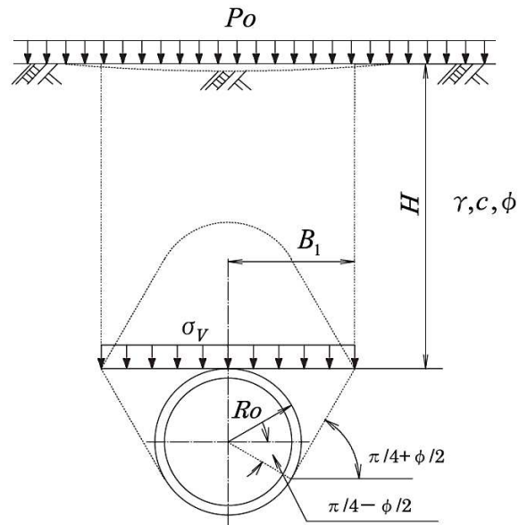
図 2.2.3.2.1-1 均一地盤における緩み土圧
