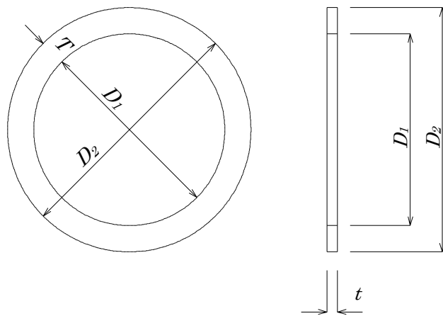
図 3.2.5.1-1 クッション材の形状
