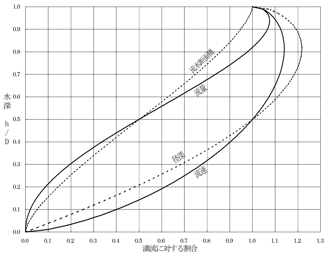
図 2.1.2-1 水力特性曲線
